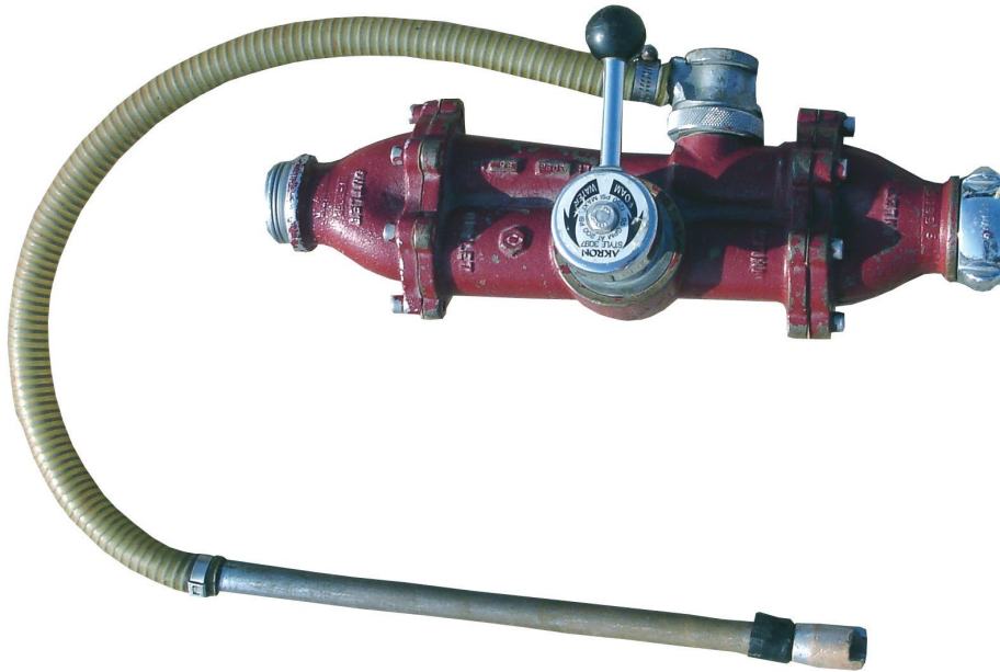
Figura 6.4: indicador de derivación
